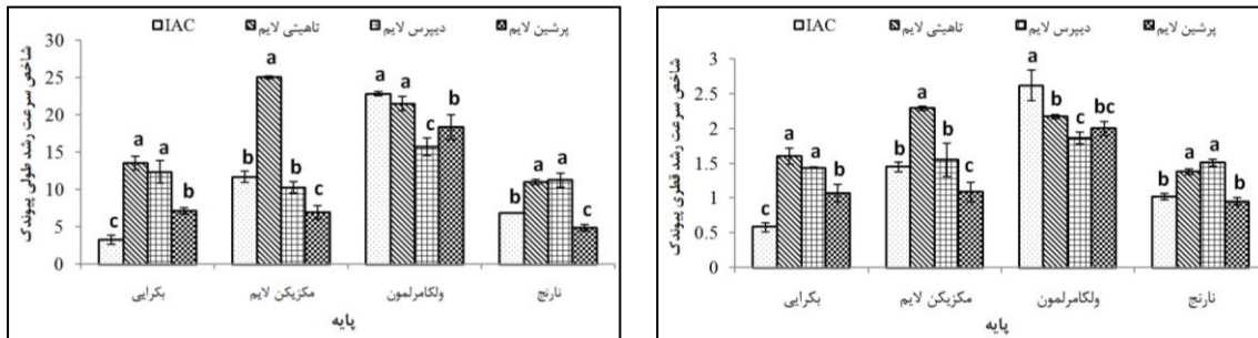
شکل ۲- مقایسه شاخص سرعت رشد طولی و قطری پیوندک ژنوتیپ‌های مختلف پرشین لایم روی چهار پایه مورد بررسی
