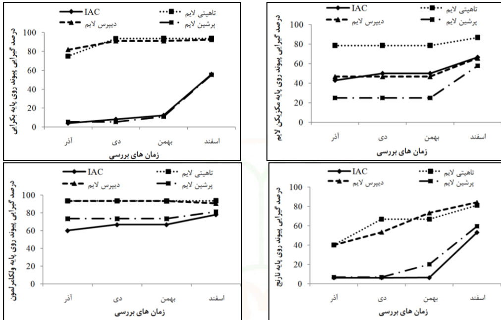
شکل ۱- روند تغییرات درصد گیرایی پیوند در پیوندک‌های مورد بررسی روی پایه‌های مختلف
